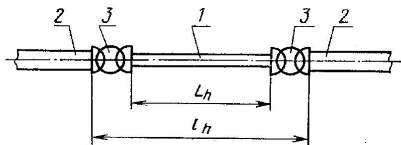
Размеры нити накала
