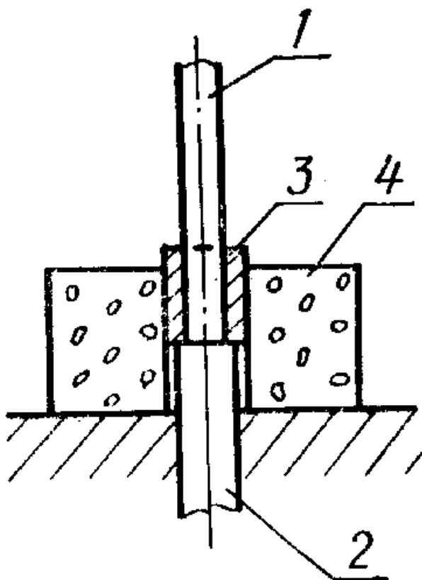
1— нить накала; 2—провод; 3—втулка после крепления; 4—пожаробезопасная подставка Черт.5
